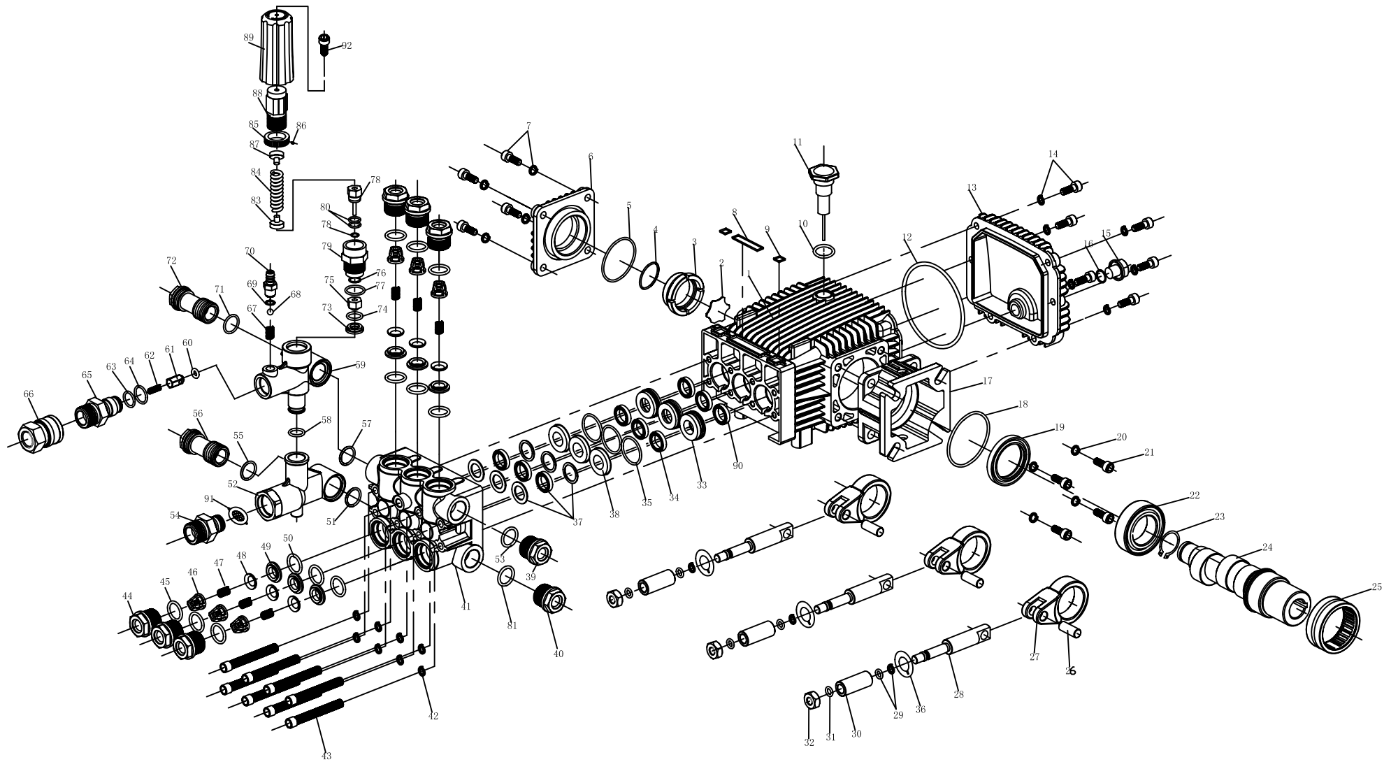
LB3WZ-15XX系列清洗机高压泵零件结构分解图
